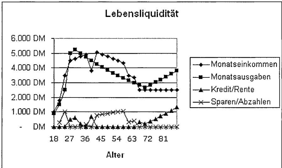
Abbildung 7: Lebensliquidität
