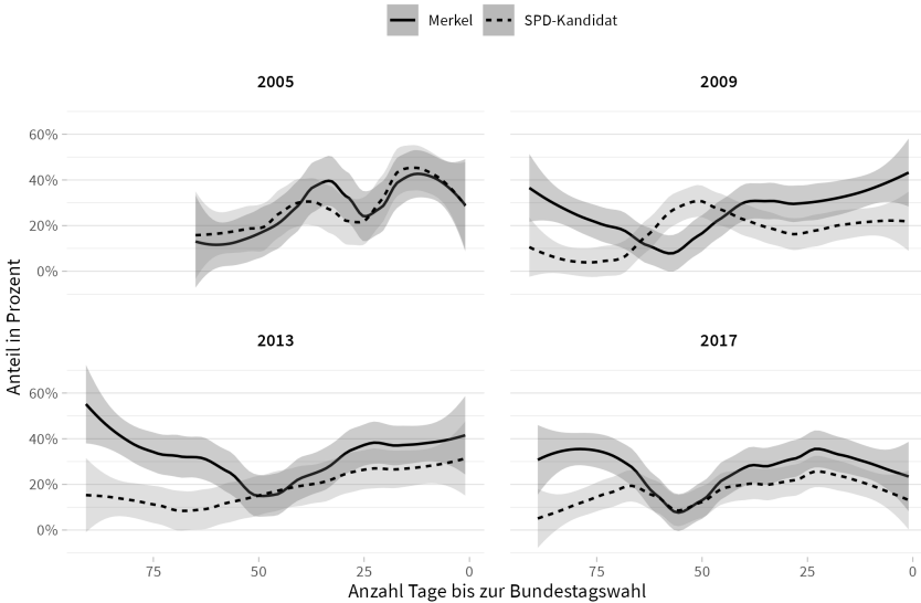
Abbildung 3: Tägliche Vorkommen der KanzlerkandidatInnen im Laufe des Wahlkampfs (Werte geglättet mittels LOWESS 1 , bw = 0,5 , die Flächen zeigen das 95-Prozent-Konfidenzintervall)
