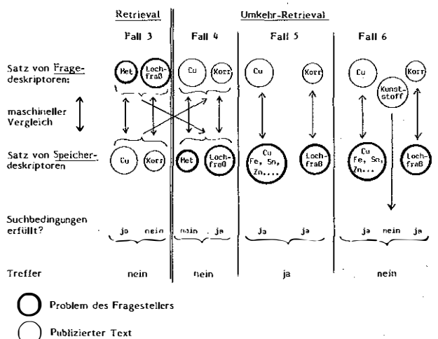
Abb. 3: Verlauf von Retrieval und Umkehrretrieval
