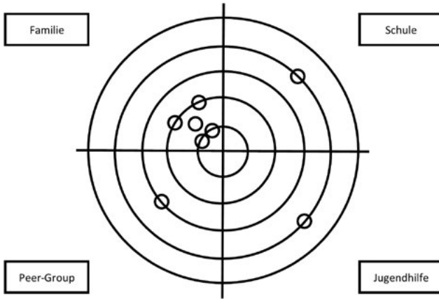
Abbildung 2: Netzwerkkarte Interviewteilnehmer_in
